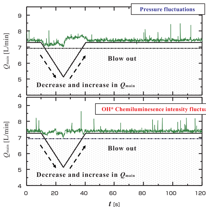
図：垂直可視グラフの平均次数を用いた吹き消えの回避 H. Gotoda et al., Physical Review Applied, vol. 7, 044027, 2017.
