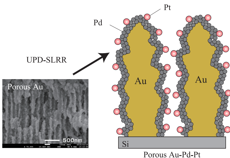
図：第三世代の Au-Pd-Pt 触媒
