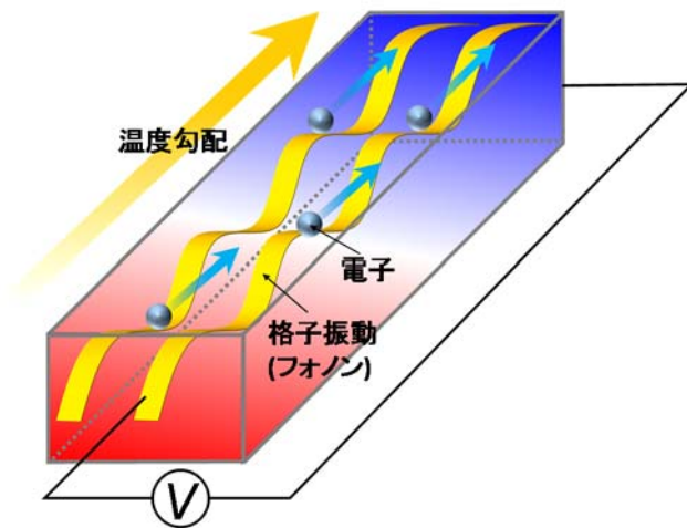
図1: フォノンドラッグ効果の概念図。結晶中の温度勾配により格子振動 (フォノン) が高温から低温に伝わる。フォノンは、電子—格子相互作用を通じて電子を運ぶことが可能であり、また電子と同様に高温側から低温側に移動する性質をもつため、通常の熱電効果に重畳する形で温度勾配の方向に電圧を発生させることができる。
