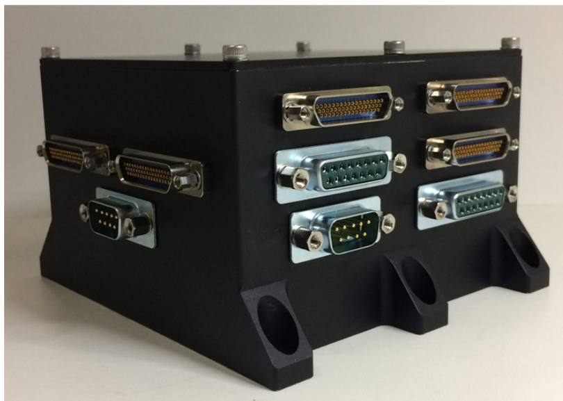
図1：IDEA OSG 1 主搭載計算機
