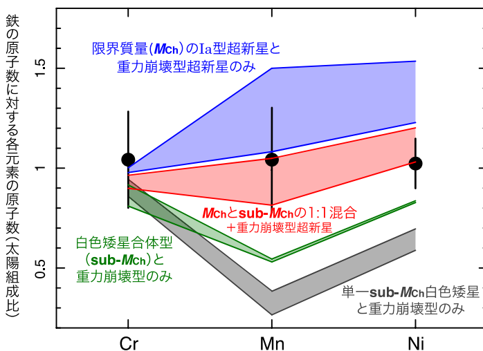
図3：ASTRO-H 衛星の観測から求められた鉄属元素の組成比 (黒丸)。青、赤、緑、灰色の色の範囲は、Ia 型超新星と重力崩壊型超新星の組み合わせを考えた場合の組成比。
