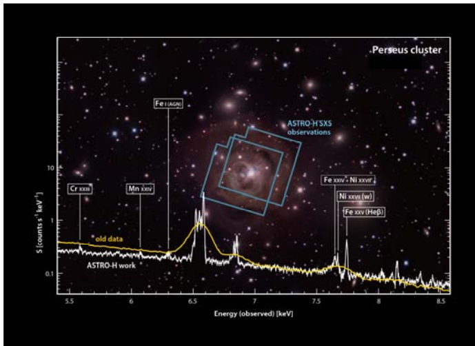
図1：ペルセウス座銀河団の可視、X線合成画像と、ASTRO-H衛星により得られたペルセウス座銀河団中心部のX線スペクトル。青は観測領域、黄色はASTRO-H衛星以前に得られていたX線スペクトル。クレジット：JAXA/Ken Crawford (Rancho Del Sol Observatory)
