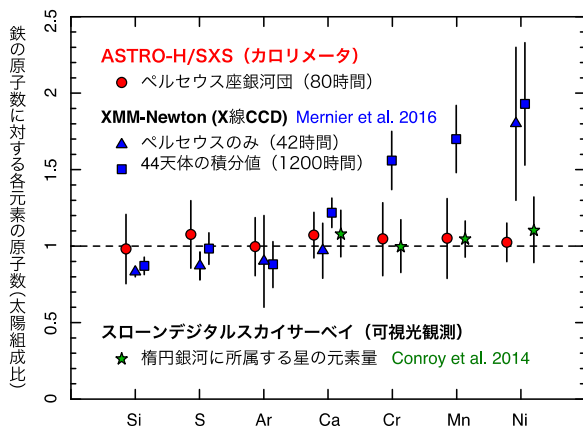
図2：ASTRO-H 衛星により観測されたペルセウス座銀河団中心部の銀河団ガスの元素組成比 (赤丸)。青のデータは、これまでの X 線天文衛星に搭載されていた CCD 検出器による結果。緑の星印は可視光観測による楕円銀河に所属する星の元素量。
